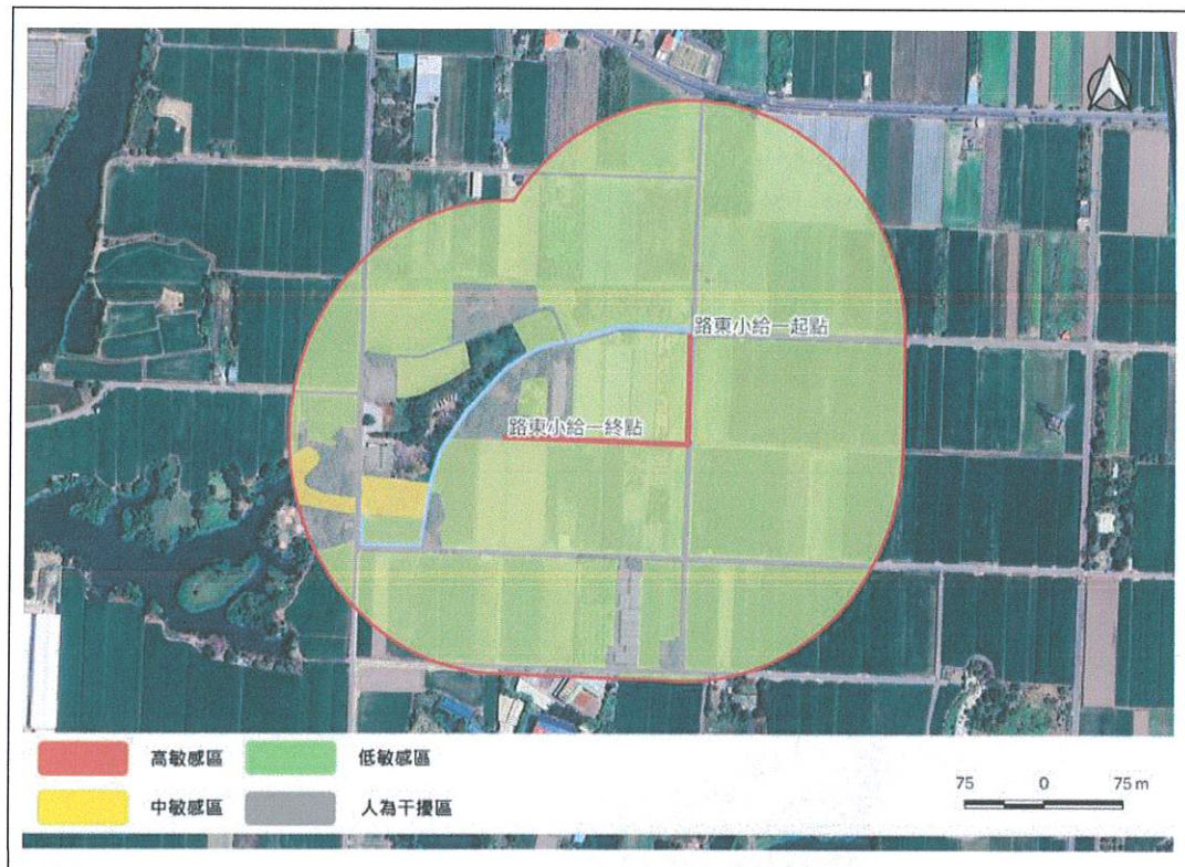
圖 5. 吉貝耍小給一之一等 4 線改善工程生態敏感區圖。
