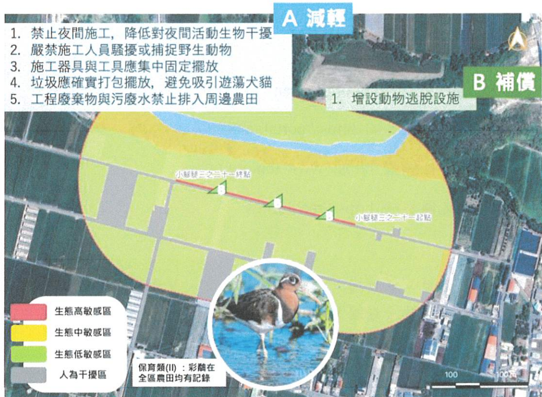
圖 7. 西勢小排二之四等 9 線改善工程生態關注區域圖。
