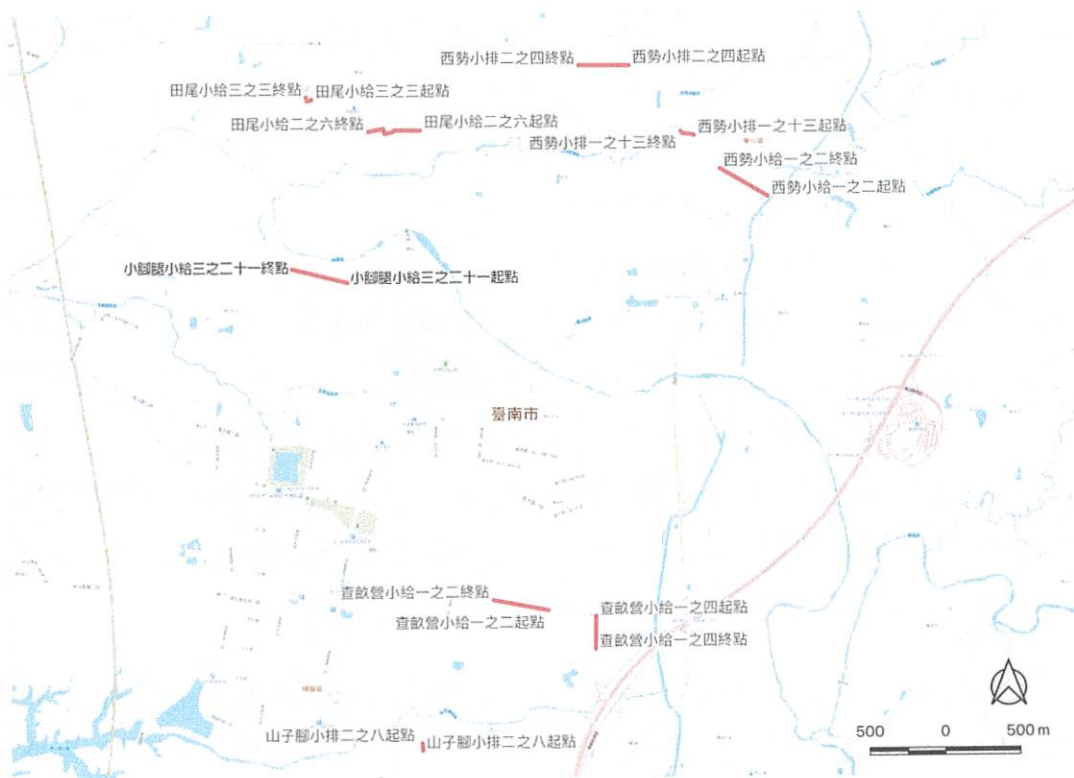
圖 1. 西勢小排二之四等 9 線改善工程位置圖(紅線處)
