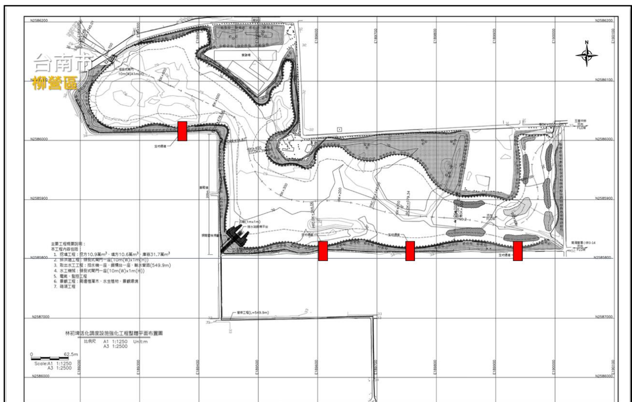
圖 3-4-3 林初埤工區位置和生物友善通道配置圖
