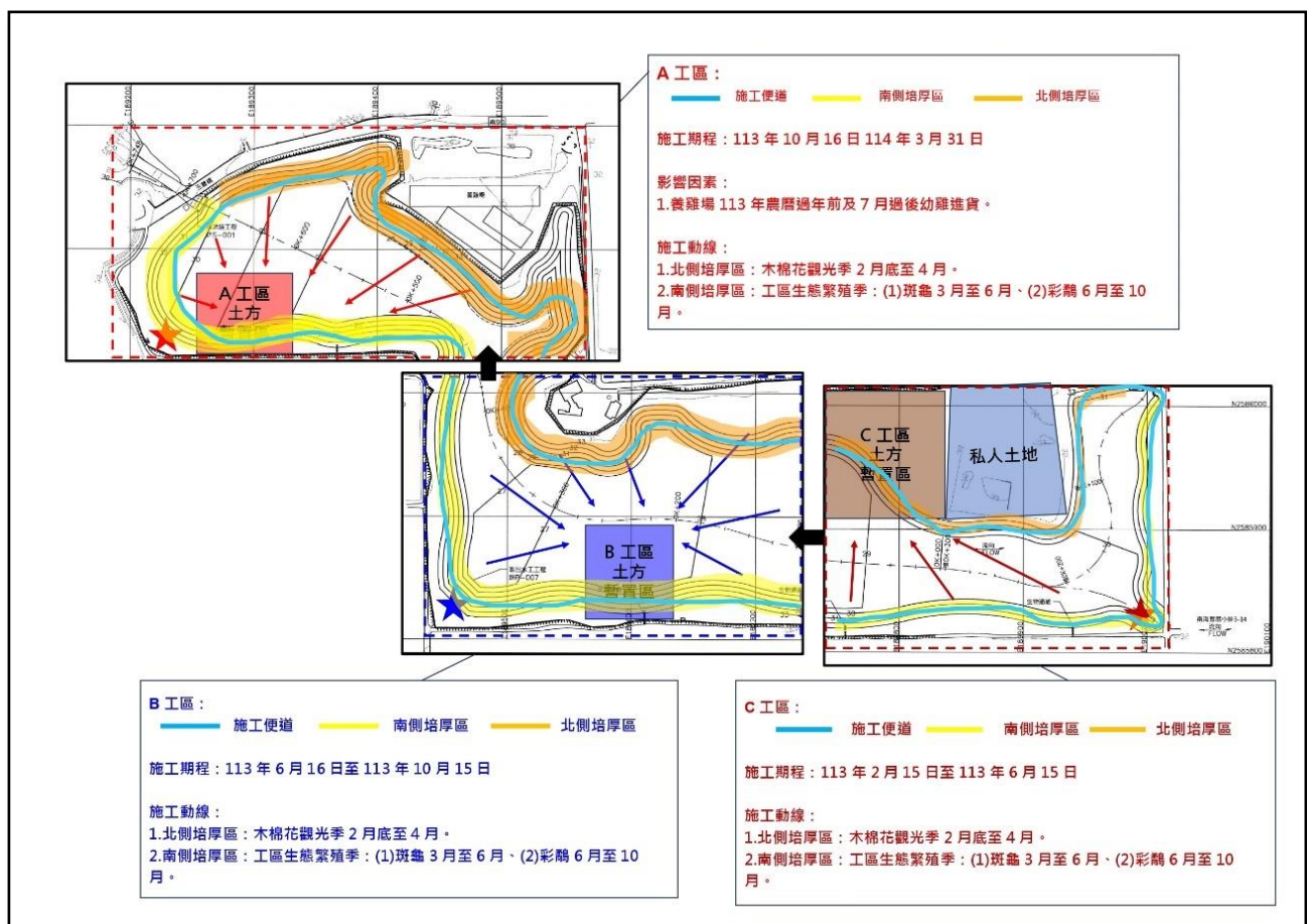
圖 3-4-5 林初埤工區臨時設施配置圖
